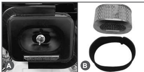
Рис. 17 Воздушный фильтр
